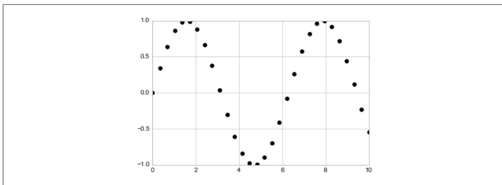
图 4-20：散点图
