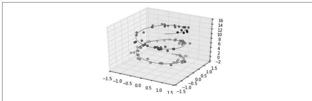
图 4-93：三维点线图
