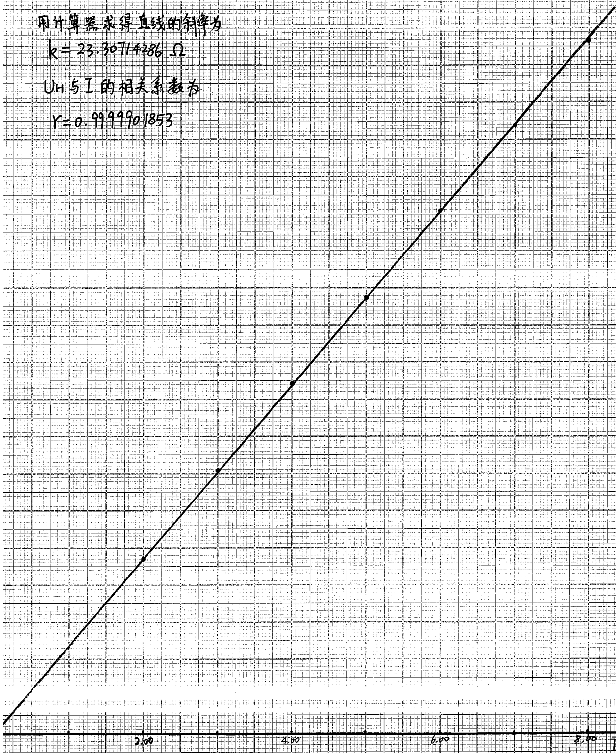
霍尔片输出电压 U_H 与输入电流 I 的关系曲线
