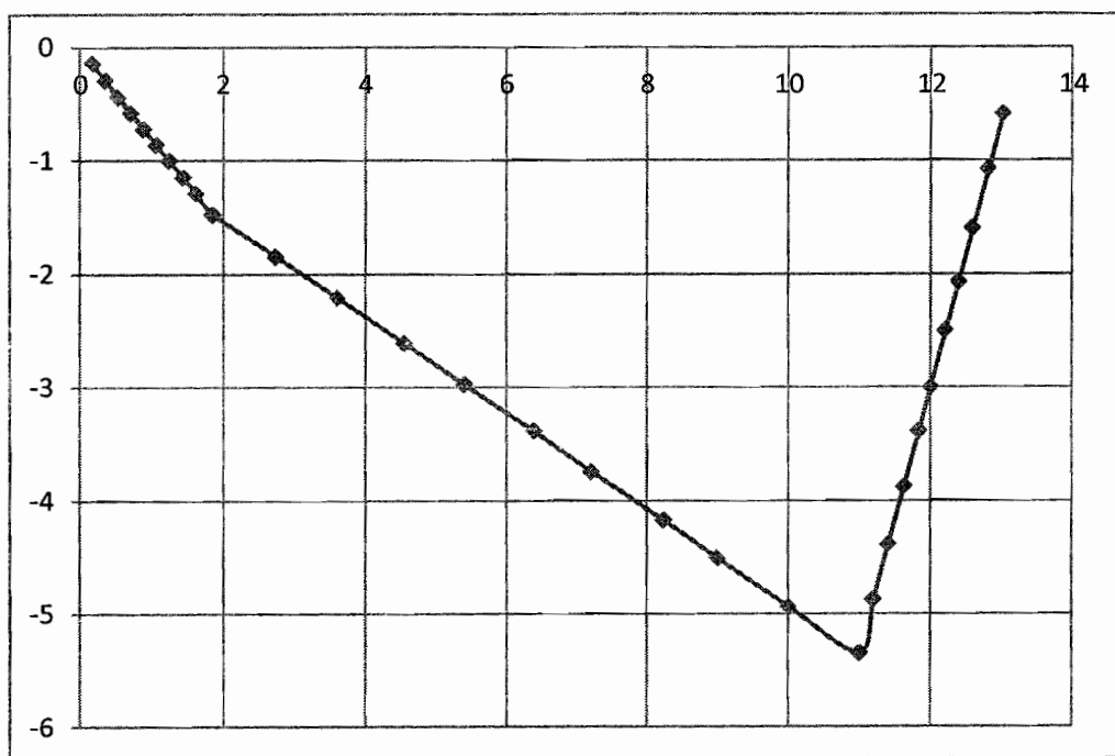
实验 U-I 曲线
