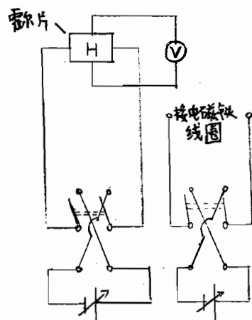
图1 实验1、2、4电路
